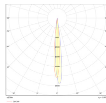
Beam Angle:15°
