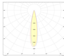
Beam Angle:15°
